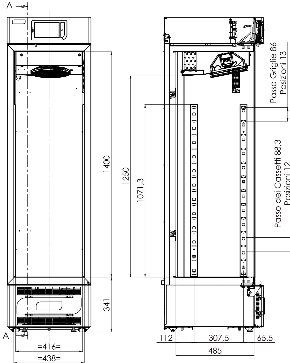
SEZIONE A-A
